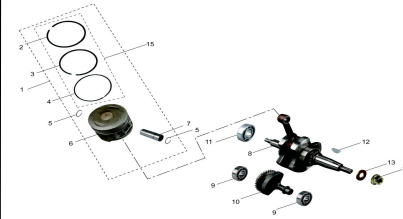
CIGÜEÑAL / PISTÓN CRANKSHAFT CONNECTING-ROD / PISTON
