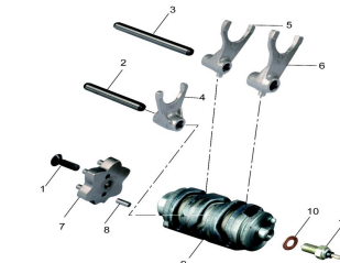
MECANISMO DE CAMBIO GEARSHIFT MECHANISM
