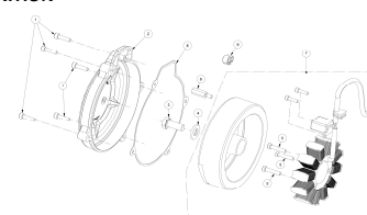
ENCENDIDO IGNITION
