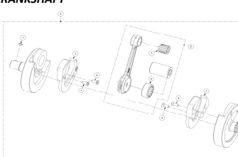
CIGUEÑAL CRANKSHAFT
