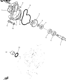
BOMBA AGUA WATER PUMP
