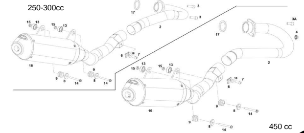
TUBO DE ESCAPE EXHAUST
