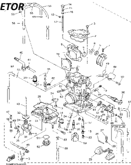
CARBURADOR CARBURETOR
