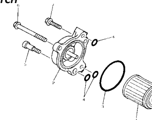
EMBRAGUE CLUTCH
