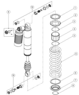
AMORTIGUADOR TRASERO REAR SHOCK
