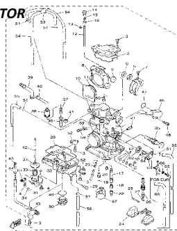
CARBURADOR CARBURETOR
