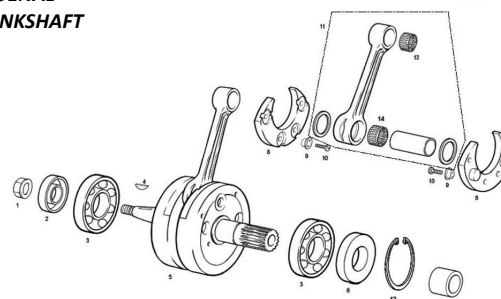
CIGÜEÑAL CRANKSHAFT
