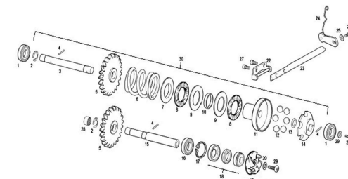
CENTRÍGUGO-BOMBA AGUA CENTRIFUGAL-WATER PUMP
