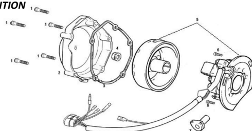
ENCENDIDO IGNITION
