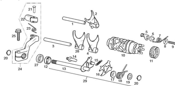
SELECTOR CAMBIO SHIFT CAM
