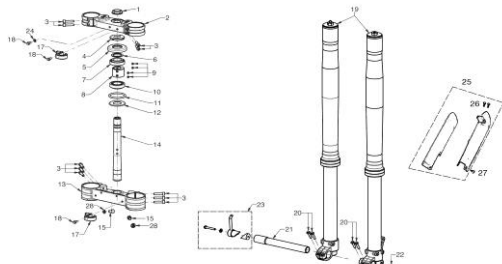
SUSPENSIÓN DELANTERA FRONT SUSPENSION
