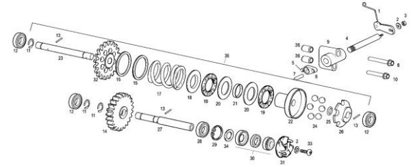
CENTRÍGUGO-BOMBA AGUA CENTRIFUGAL-WATER PUMP
