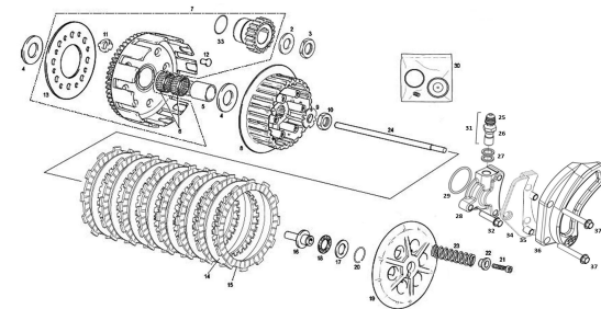
EMBRAGUE CLUTCH
