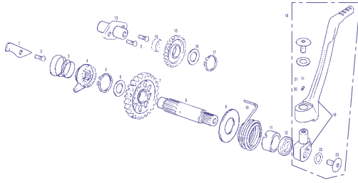
Conjunto pedal arranque / Kickstart set CASCAS WILD H.P.
