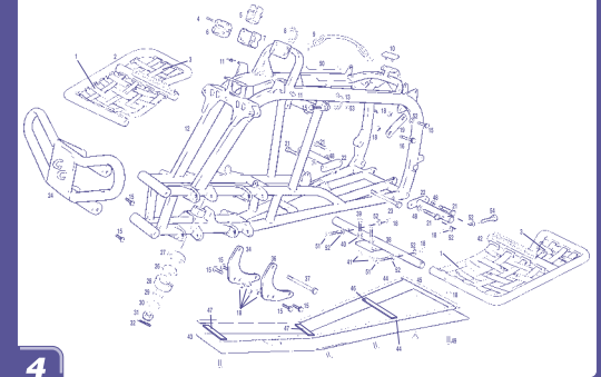
Chasis / Frame GASGAS WILD H.P.
