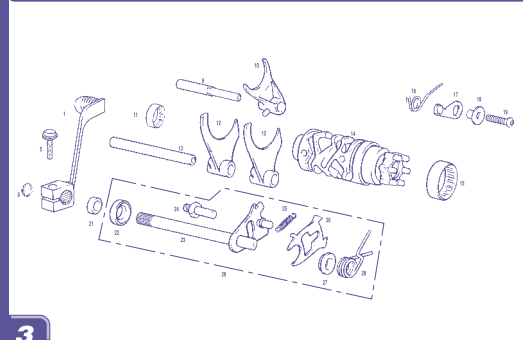
Selector cambio / Shift cam CASCAS WILD H.P.
