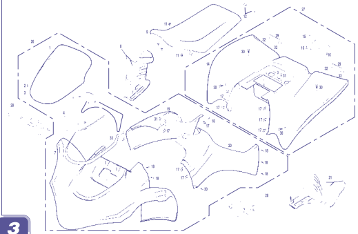
Plásticos / Plastics GASGAS WILD H.P.
