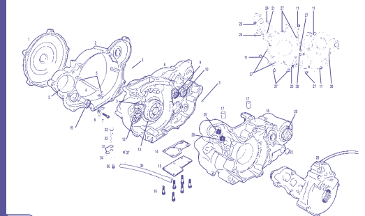
Cárter izquierdo / Left crankcase CASCAS WILD H.P.
