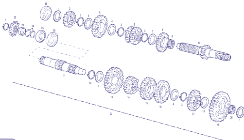
Engranajes cambio / Gear set CASCAS WILD H.P.
