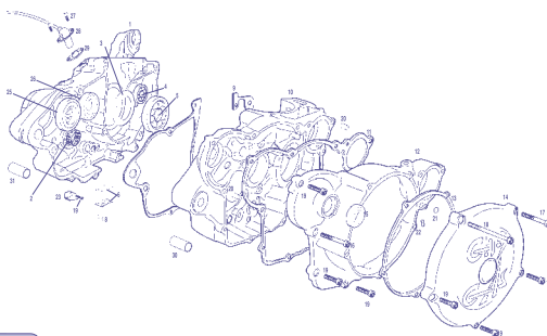
Cárter derecho / Right crankcase CASCAS WILD H.P.
