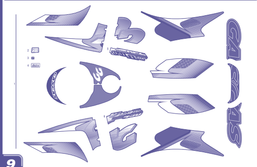
Adhesivos / Decals GASCAS WILD H.P.
