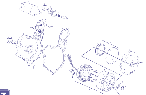
Encendido / Ignition CASCAS WILD H.P.
