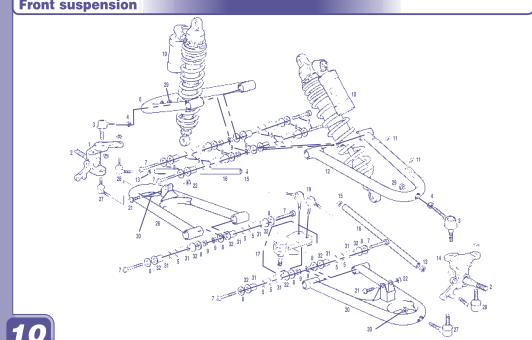
Suspensión delantera / Front suspension GASCAS WILD H.P.
