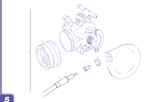
Cuerpo Mariposa / Throttle body GASGAS WILD H.P.
