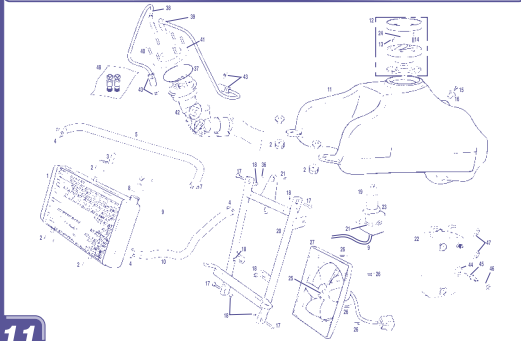
Depósito / Fuel tank GASCAS WILD H.P.
