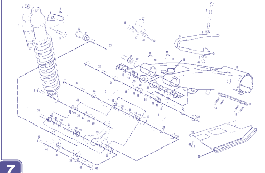
Basculante / Swingarm GASGAS WILD H.P.
