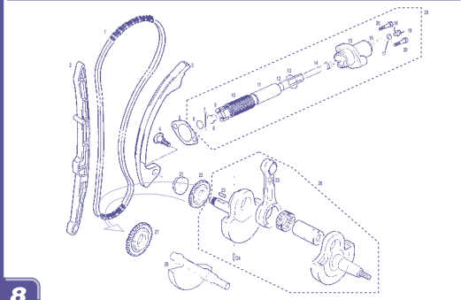
Cigüeñal / Crankshaft GAS GAS WILD H.P.
