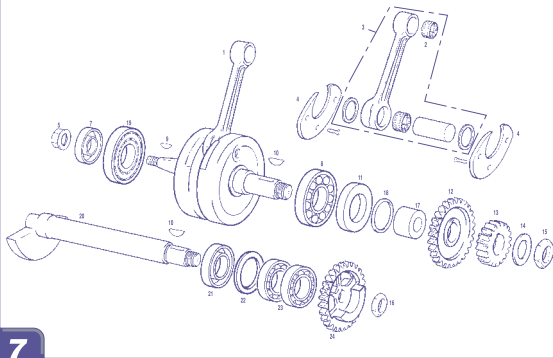
Cigüeñal / Crankshaft GAS GAS WILD H.P.
