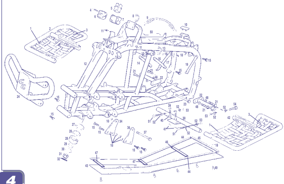
Chasis / Frame CASCAS WILD H.P.
