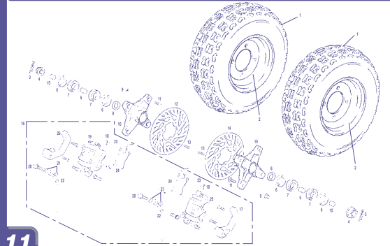
Rueda delantera / Front wheel CASCAS WILD H.P.
