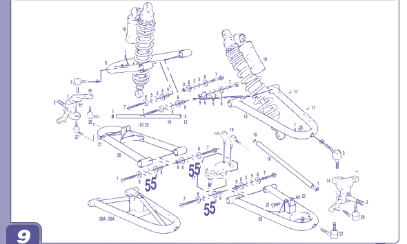
Suspensión delantera / Front suspension CASCAS WILD H.P.
