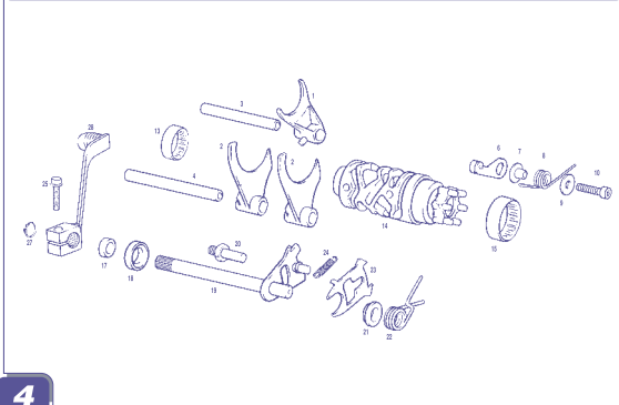
Selector cambio / Shift cam GAS GAS WILD H.P.
