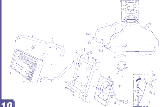
Depósito / Fuel tank CASCAS WILD H.P.
