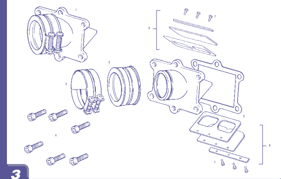
Caja láminas / Reed valve GAS GAS WILD H.P.
