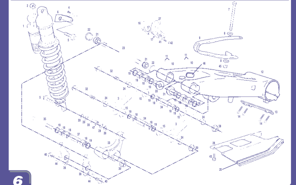
Basculante / Swingarm CASCAS WILD H.P.
