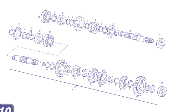
Engranajes cambio / Gear set GAS GAS WILD H.P.
