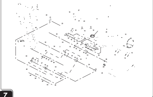
Basculante / Swingarm CASGAS WILD HP
