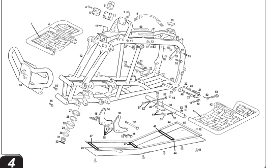
Chasis / Frame CASGAS WILD HP
