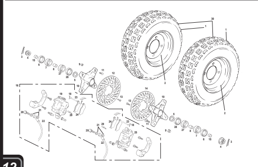
Buena delantera / Front wheel GASGAS WILD HP
