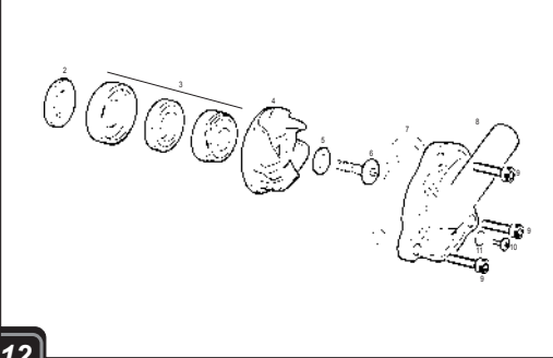
Bomba agua / Water pump GASGAS WILD HP
