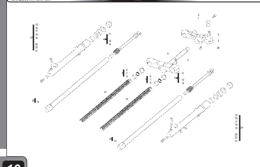
Suspension MARZOCCHI / MARZOCCHI Front Fork GASGAS EC / SM ROOKIE 05
