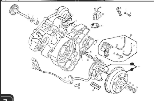
Chasis o magnético / Lyndant magneto
