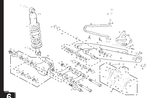
Basculante / Swingarm CASGAS EC / SM ROOKIE 05
