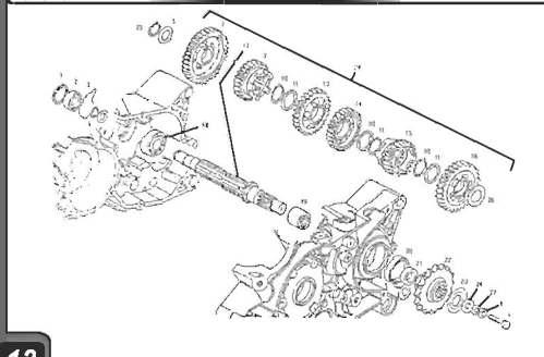
Eje secundario / Counter shaft
