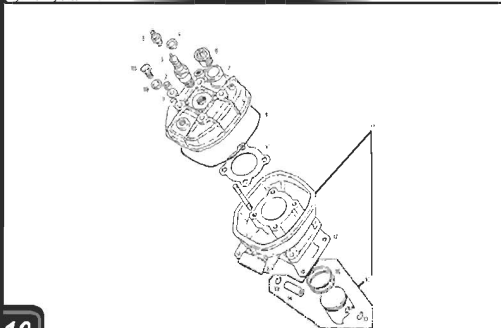
Cilindro - Cámara - Pistón / Cylinder - Cyl. head - Piston
