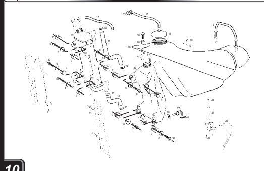
Depósito / Fuel tank GASGAS EC / SM ROOKIE 05
