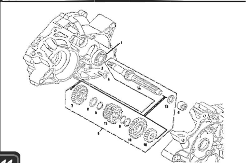
Eje primario / Main shaft
