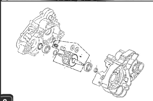
Cigüeñal / Crankshaft
