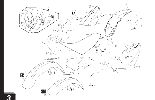
Plásticos / Plastics CASGAS EC / SM ROOKIE 05
