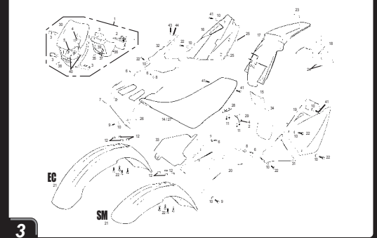
Plásticos / Plastics CASGAS EC / SM ROOKIE 05
