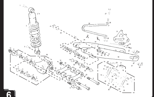
Basculante / Swingarm CASGAS EC / SM ROOKIE 05
