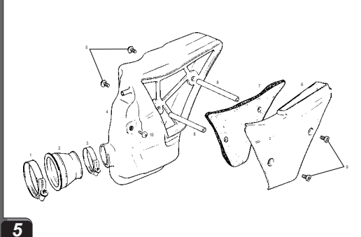
Filtro de aire / Air filter CASGAS EC / SM ROOKIE 05
