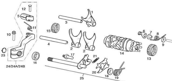
SELECTOR CAMBIO SHIFT CAM
