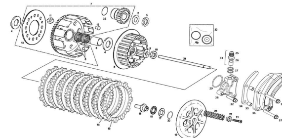
EMBRAGUE CLUTCH
